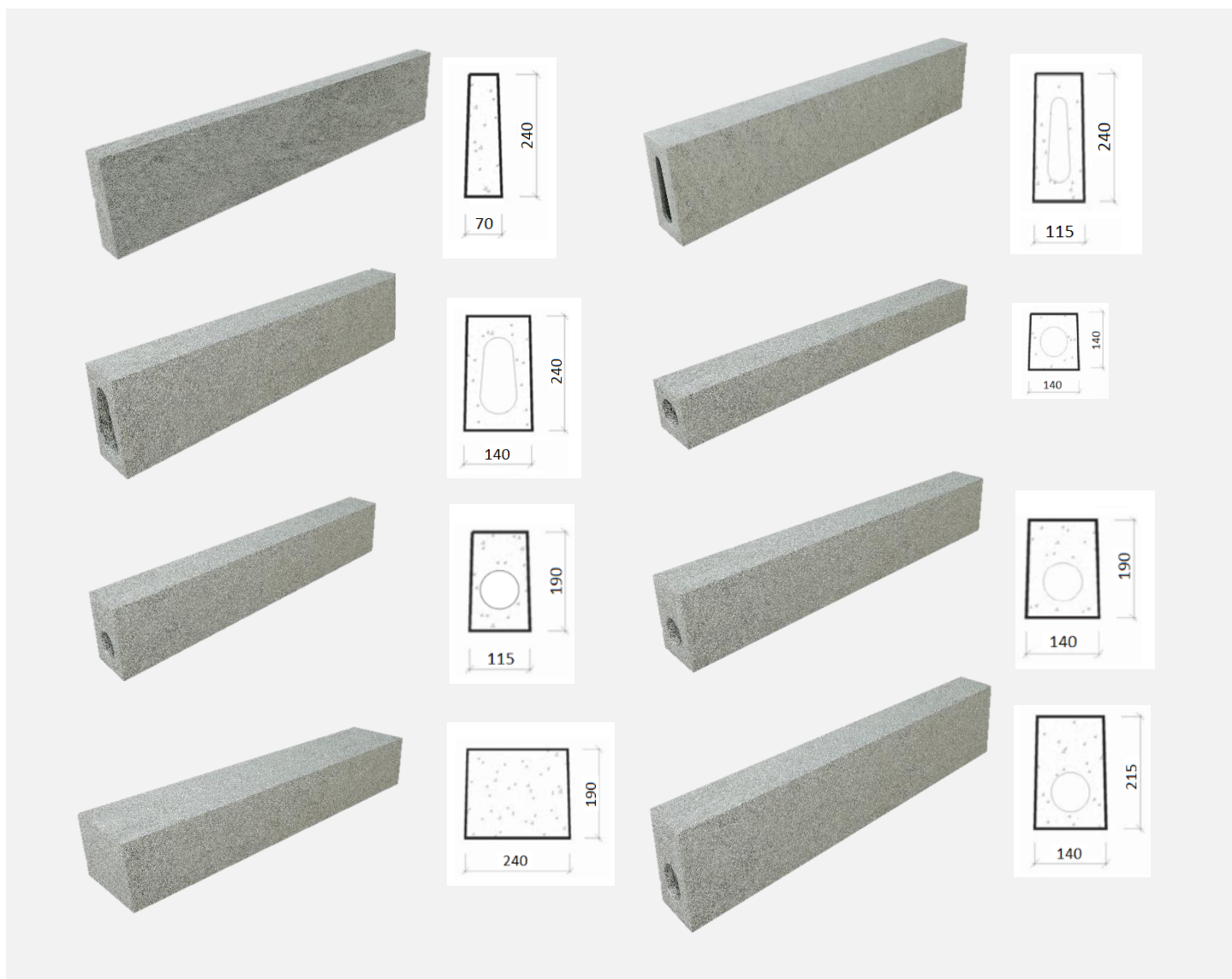
Obr 1. – Překlady a jejich řezy jednotlivými typy překladů
