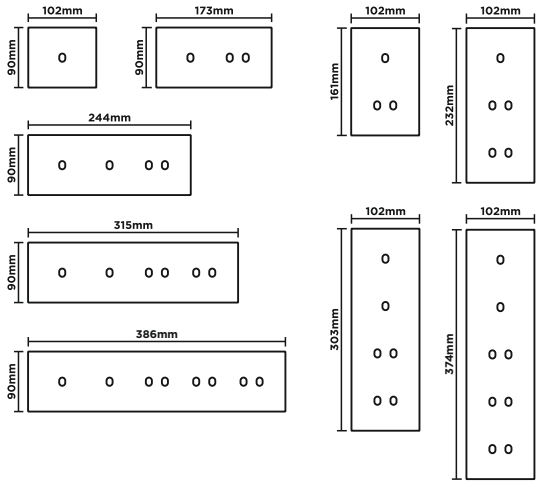
Násobnosti a rozměry rámečků
