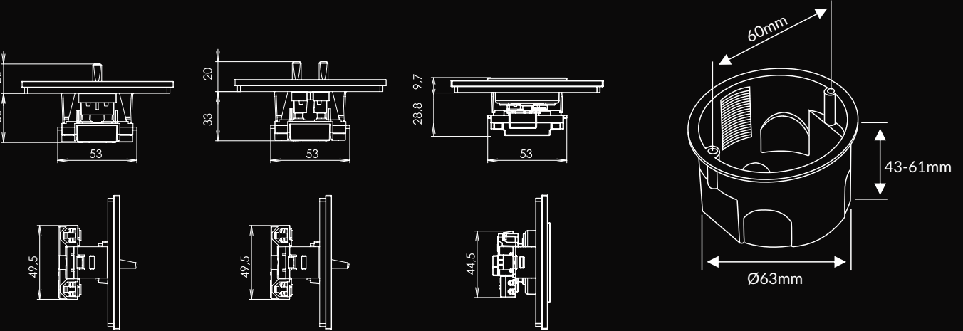
Montáž do standardních elektroinstalačních krabic Ø60mm (jednoduchých i vícenásobných, modulární pro běžné a duté stěny).
