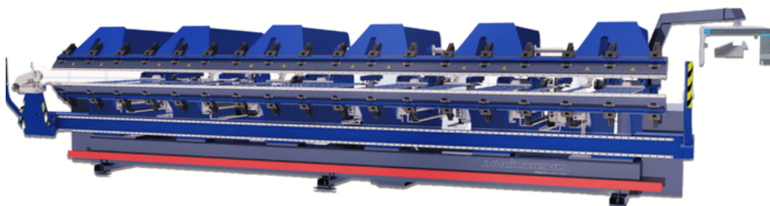
Automatická ohýbací linka VARIOBEND
