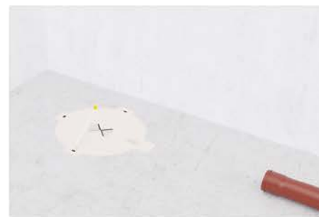
3. Montážní šablonu orientovat ve směru odtoku a vyznačit otvory pro vrtání
